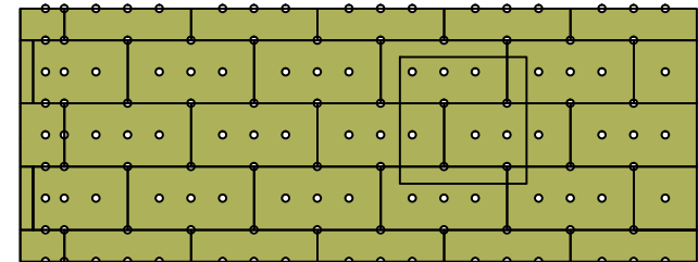
Kotvenie nad 20 m výšky
