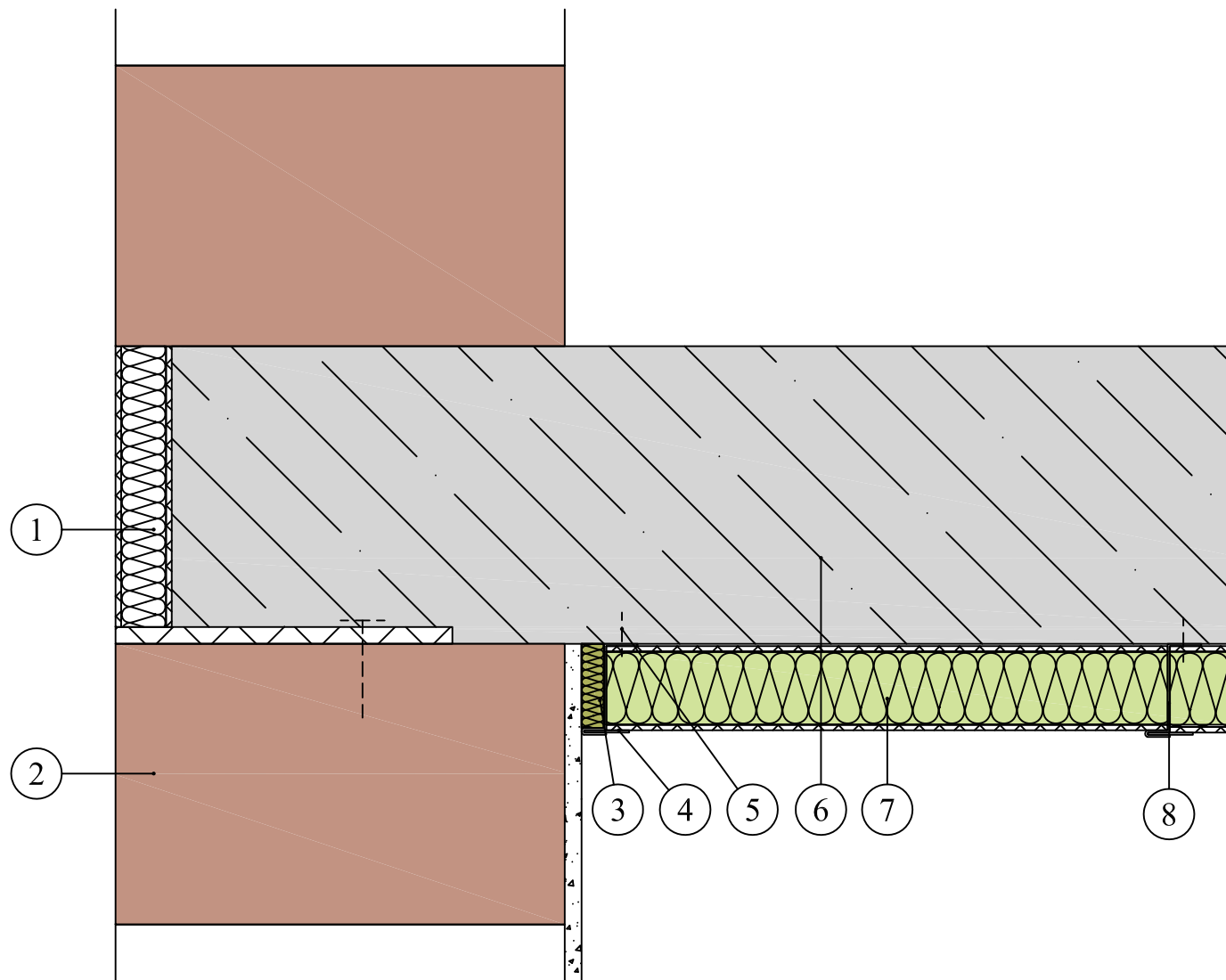
Prierez - dodatočné upevnenie a ukončenie
